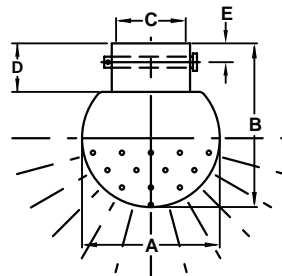
Patrón de Fondo 180°
