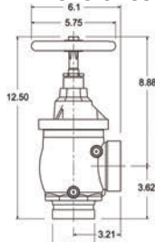
válvula de ángulo ranura x Hembra
