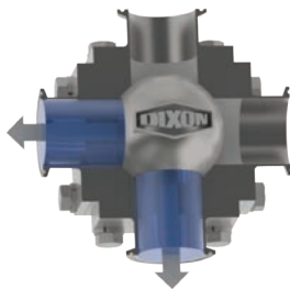
4-vías puerto 'L' posición A
