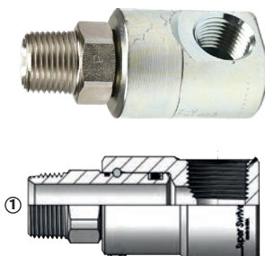
(1) Macho NPTF (2) Hembra NPTF
