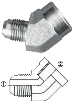
(1) Macho JIC 37° (2) Hembra NPTF
