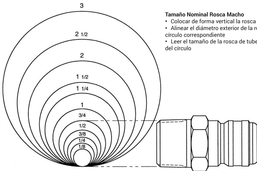
Ejemplo: 3/4 Rosca Macho (Dixon® tamaño final = 6)
