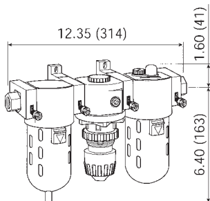
Con tazón de metal
