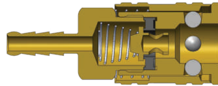
Serie-M Cople Intercambio ARO Manual (Barbas para Manguera)
