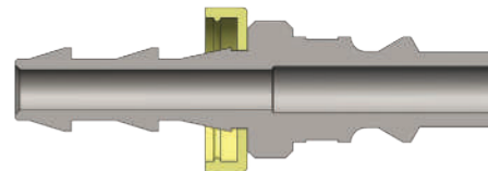
Serie-M Niple Intercambio ARO (Push-Loc)
