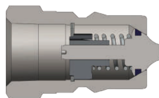
Serie-H Niple Intercambio ISO-B (Roscas Hembra)
