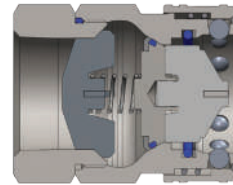
Serie-V Cople con Válvula MIL-C-51234 (Roscas Hembra)
